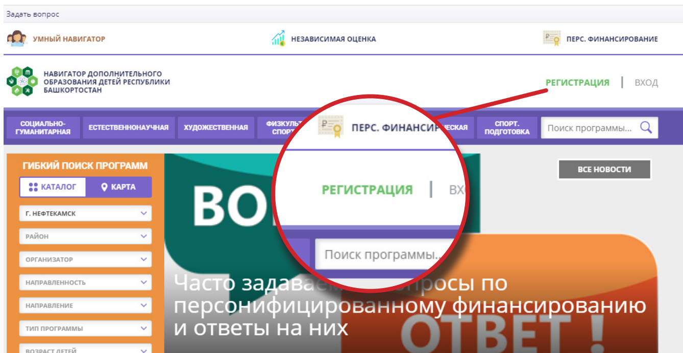
Рисунок 2. Кнопка «Регистрация»
