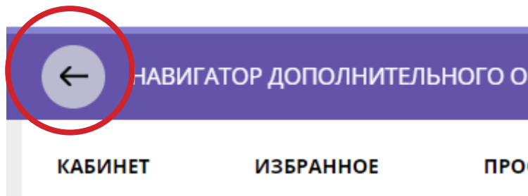
Рисунок 7. Кнопка «Назад»
