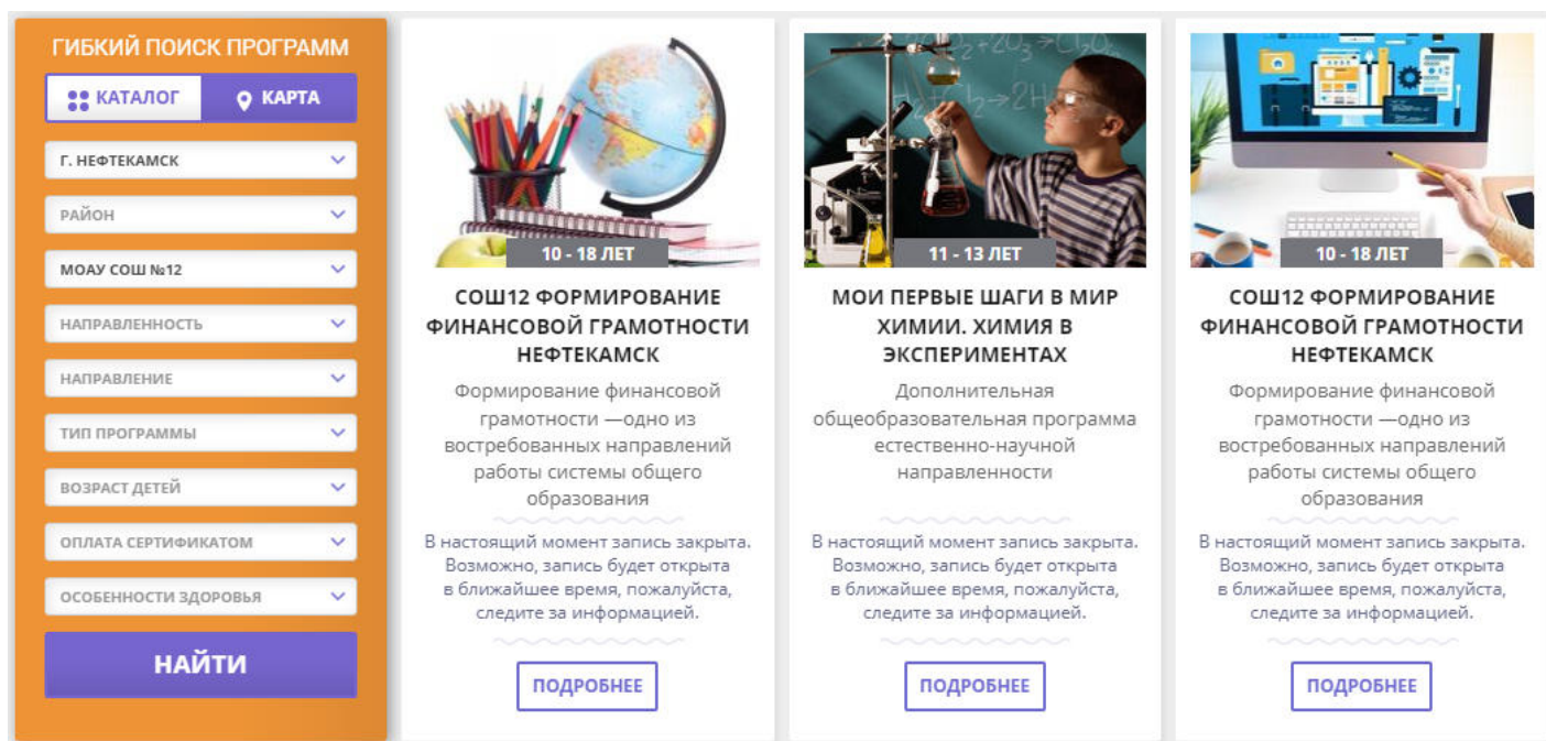
Рисунок 9. Выбор программы
